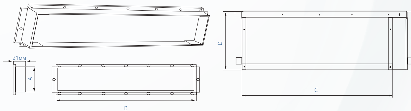
Вихід припливного повітря
